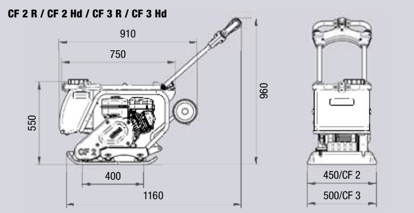
Rozměry v mm.
